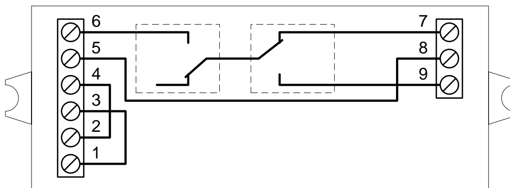
Назначение контактов.
